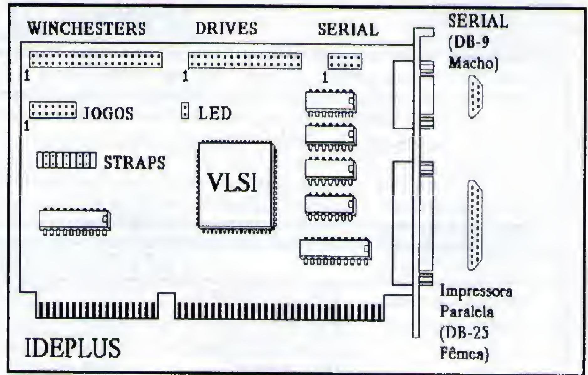
Figura 14 - placa IDEPLUS de 16 bits
